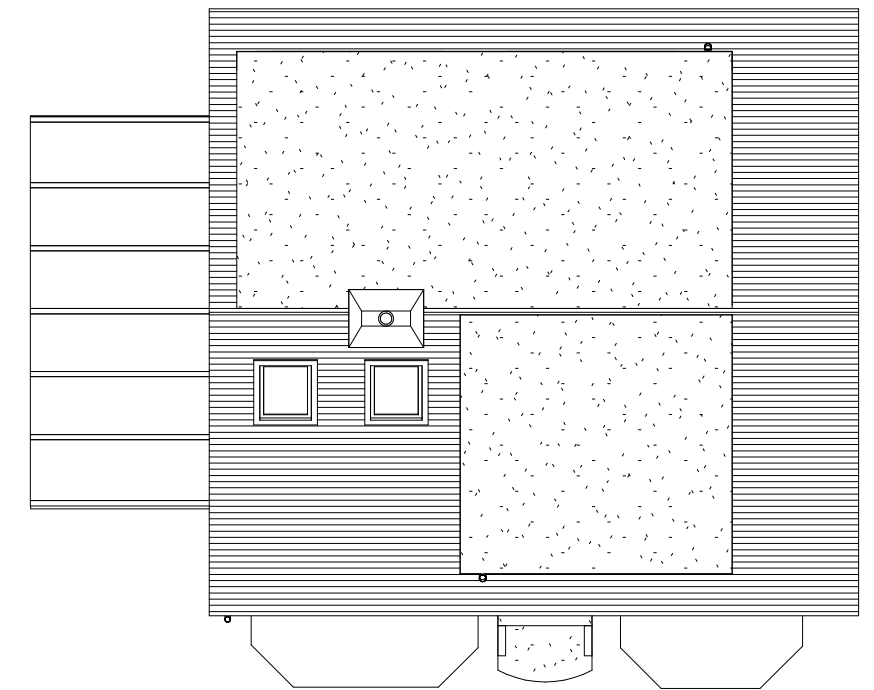
Roof Plan 1 : 100
