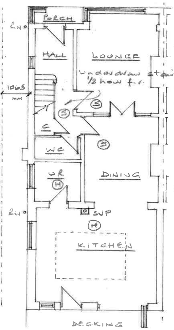
EXTG. G.F. PLAN
