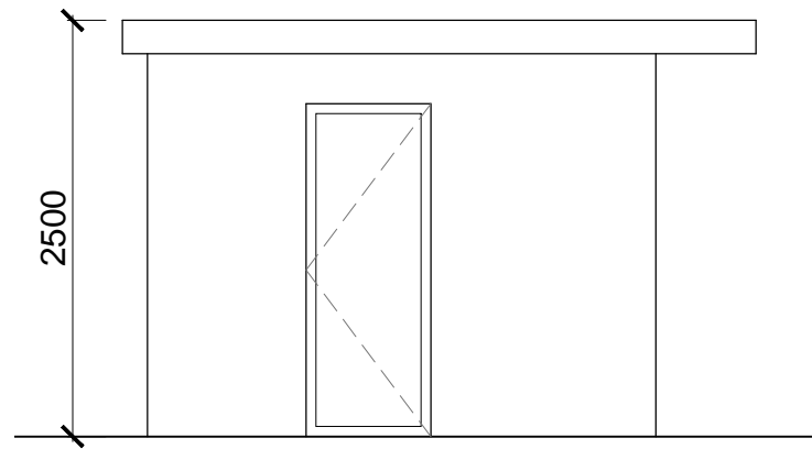
ELEVATION BB
