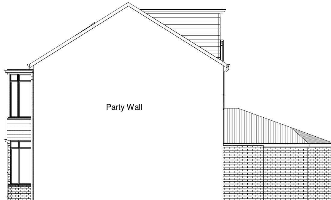
4 Side Elevation b-b 1 : 100
