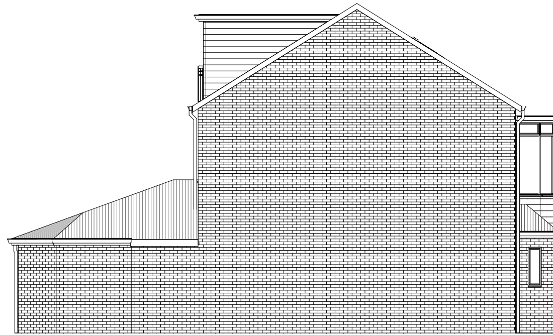
2 Side Elevation a-a 1 : 100
