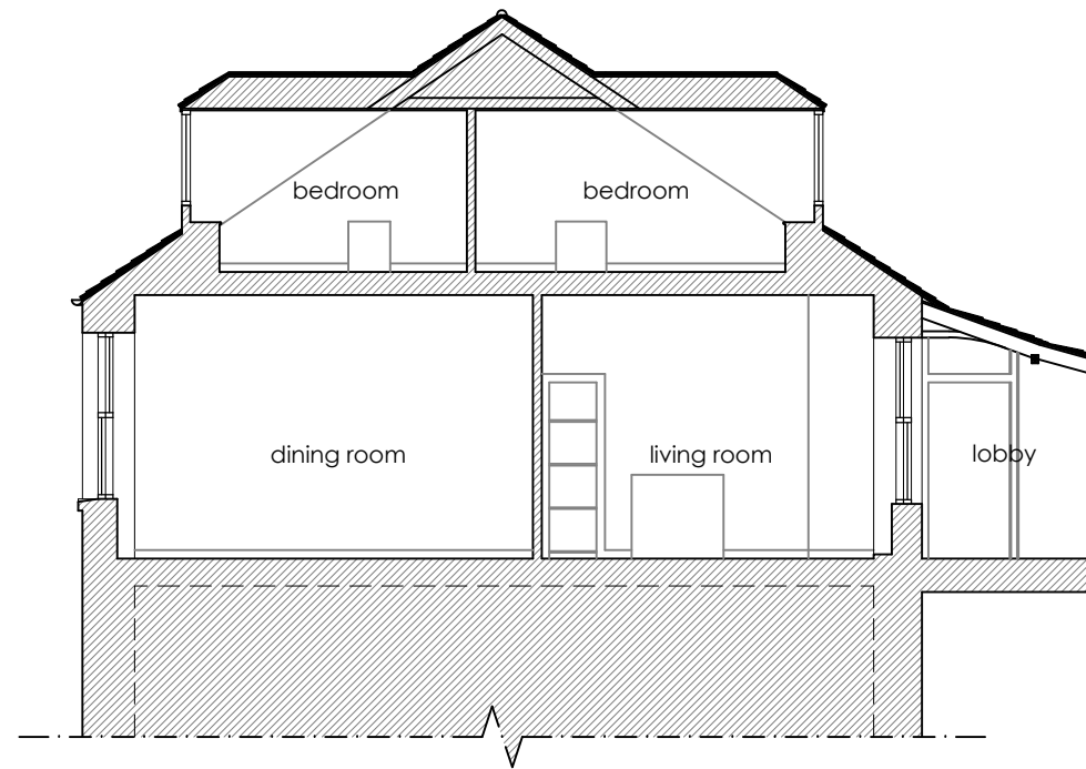
Existing Section B-B 1/100 @ A3
