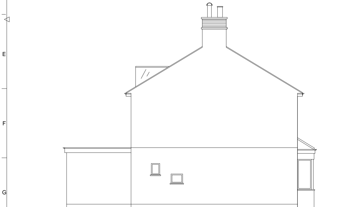
1 FRONT ELEVATION - EXISTING Scale: 1:100
