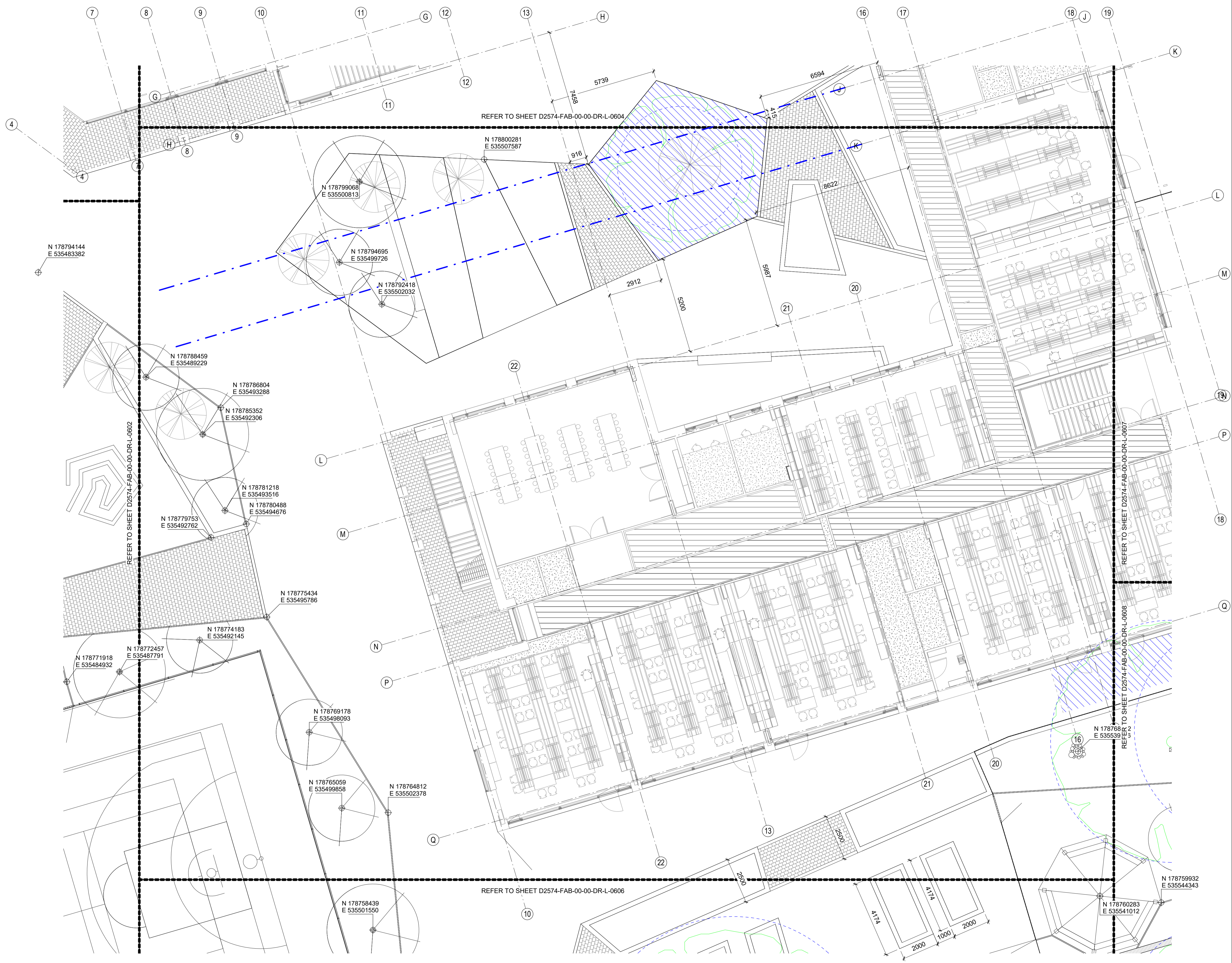
Keyplan - 0605 Scale 1 : 1500
