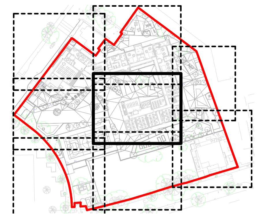
Keyplan - 0605 Scale 1 : 1500
