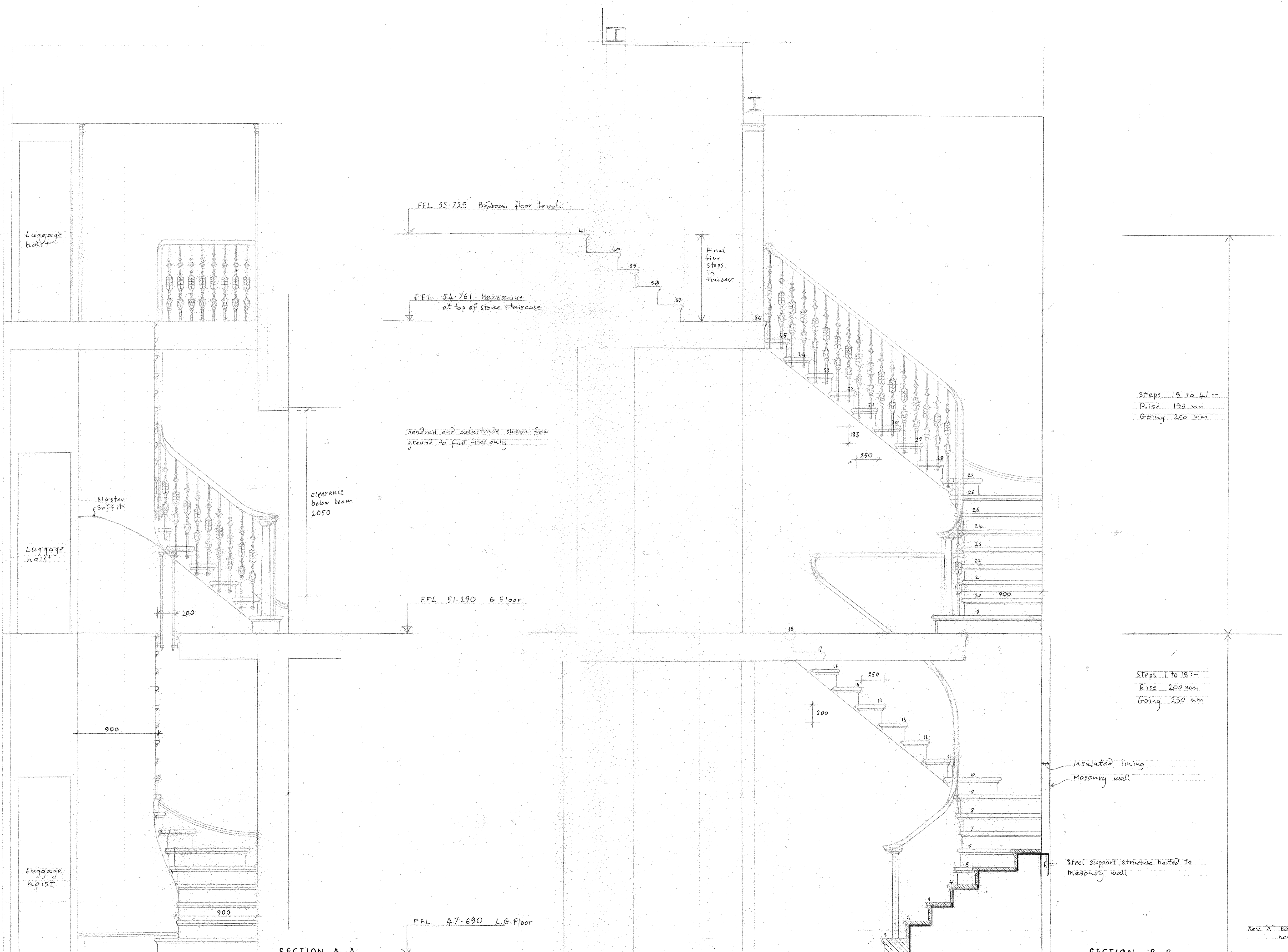
SECTION A-A
