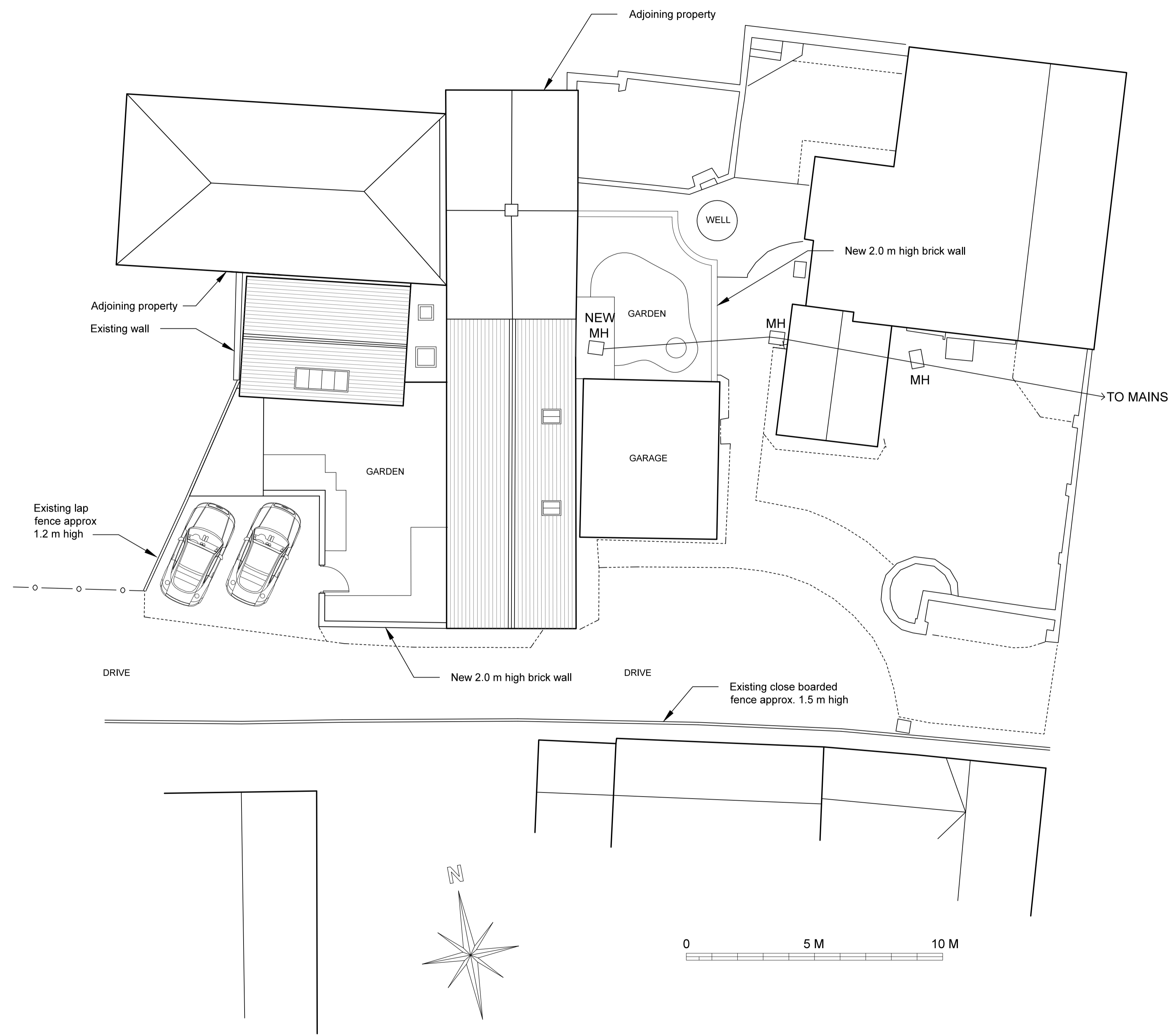
SITE PLAN 1:100 Scale
