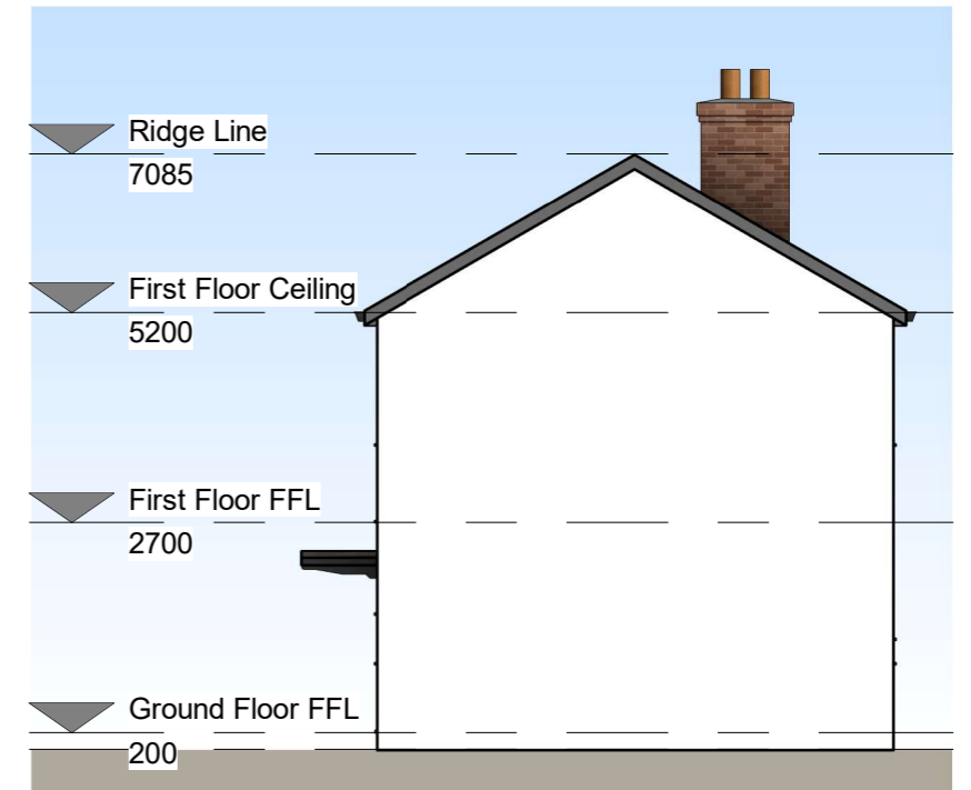
6 03 - Side Elevation 1 : 100
