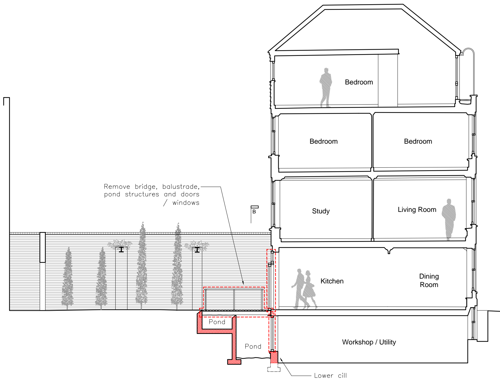
Existing Section A-A 1:100
