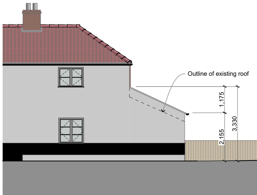
1 01 Elevation 1:100
