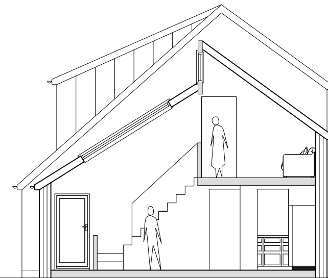
SECTION A-A 1:100
