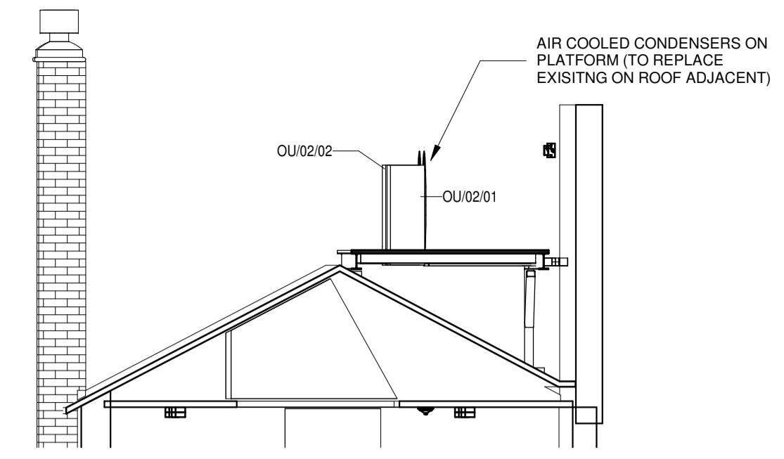
3 Air Condensers 1 : 50
