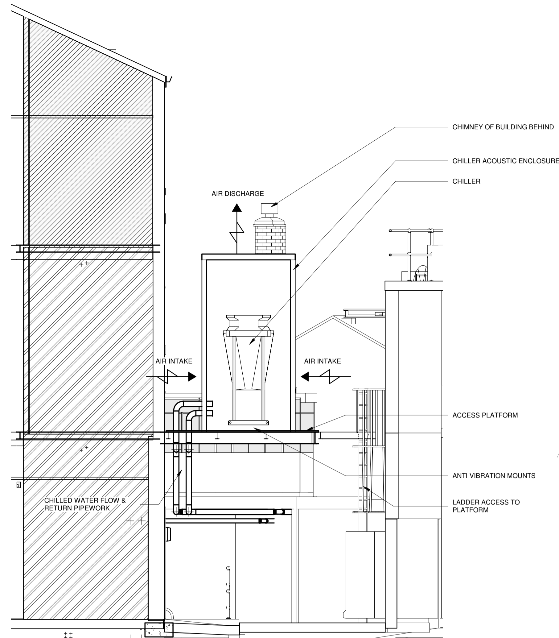
2 Chiller 1 : 50
