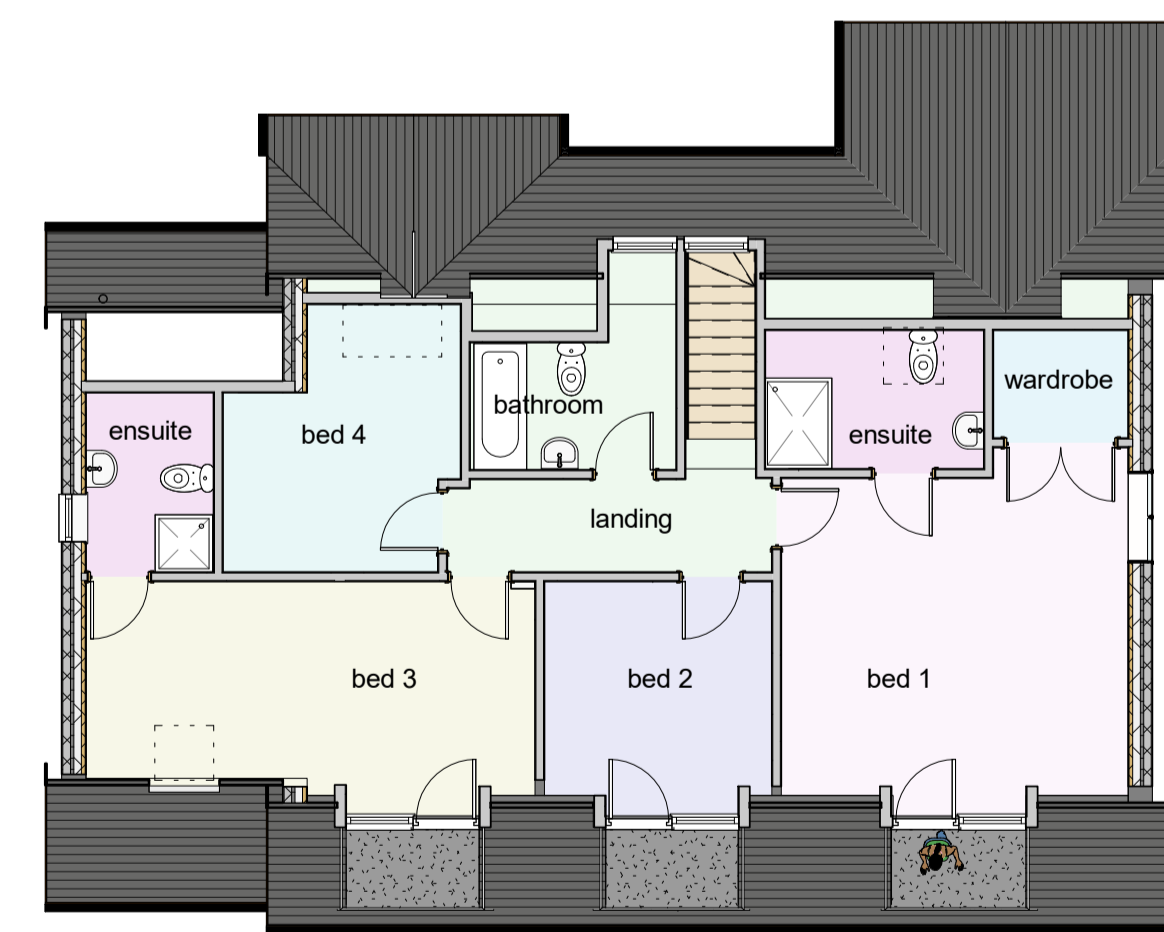
2 1_First Floor 1 : 100
