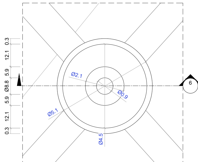
5 DETAIL Scale: 1:1
