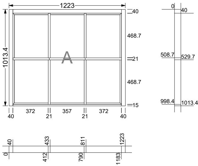
W4 Top sliding sash
