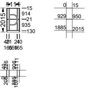
W1,W2,W3 Bottom sliding sash
