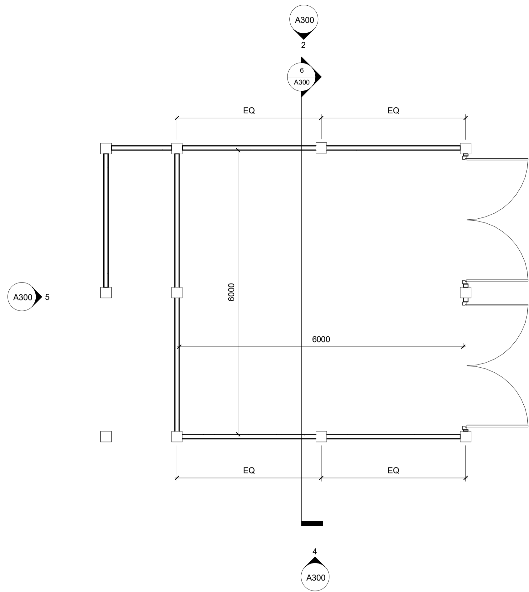
1 Plan 1 : 50
