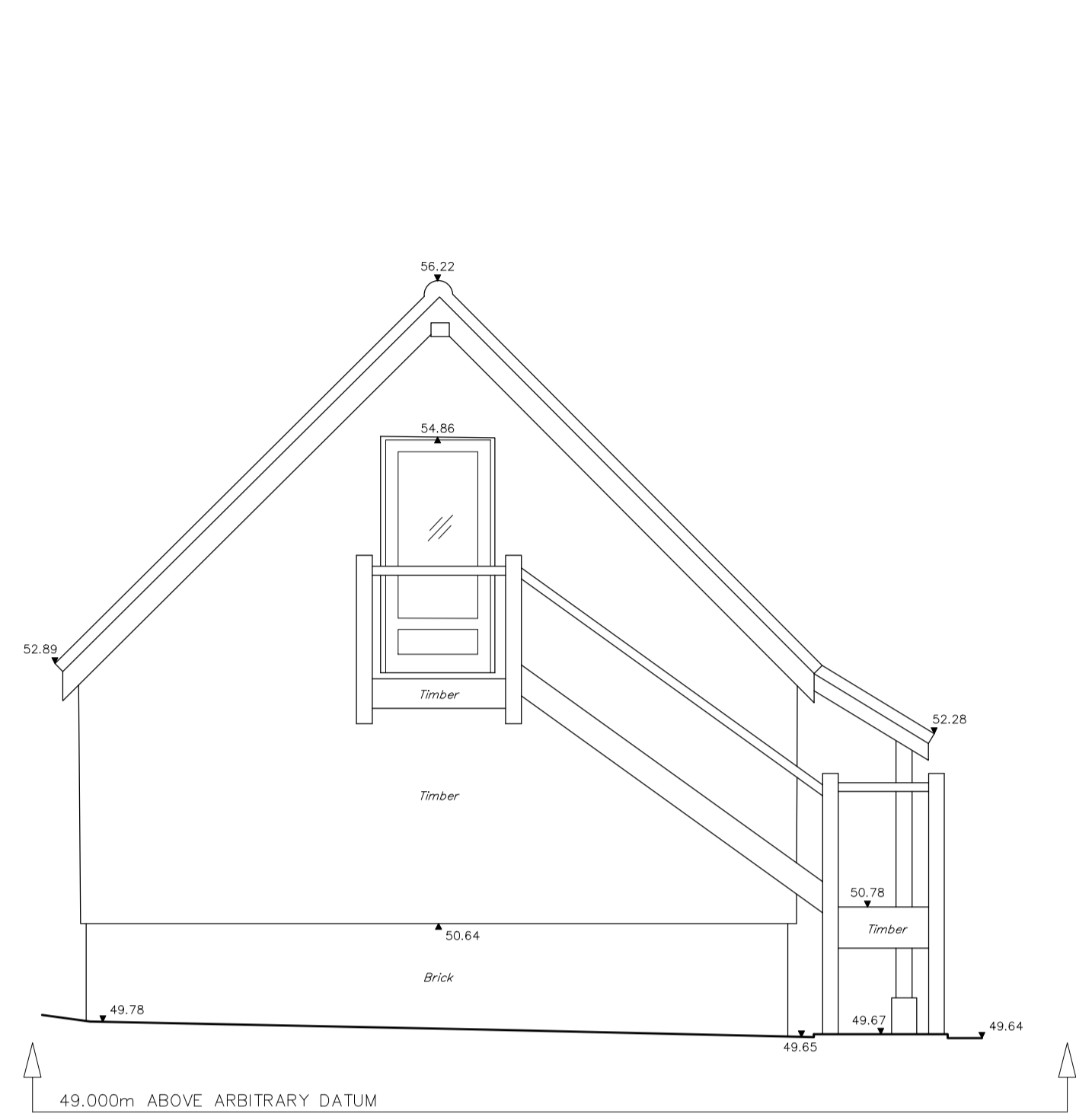
ELEVATION 1
