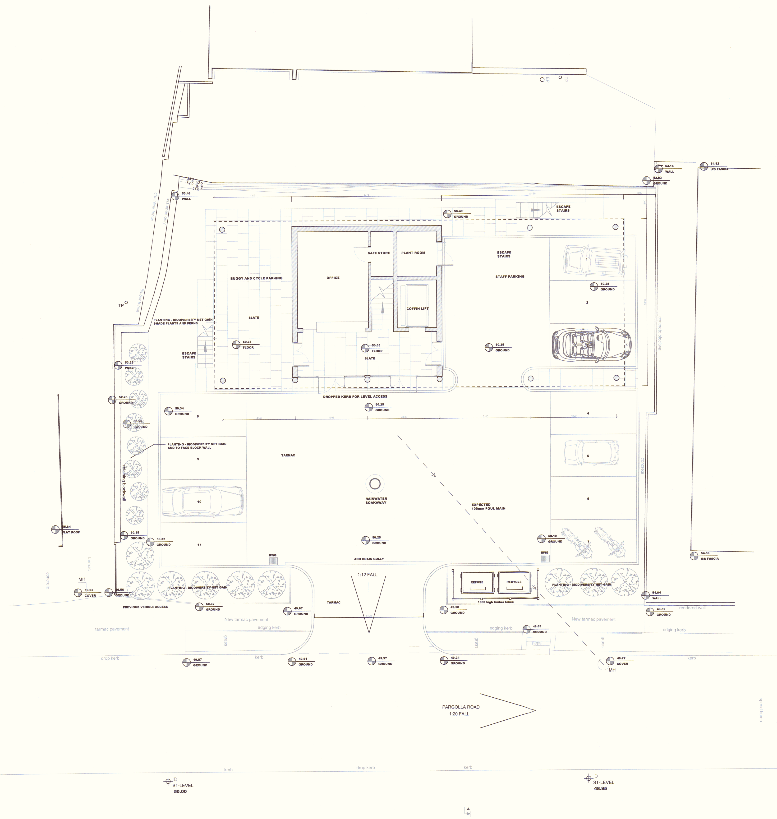
1:500 SITE PLAN
