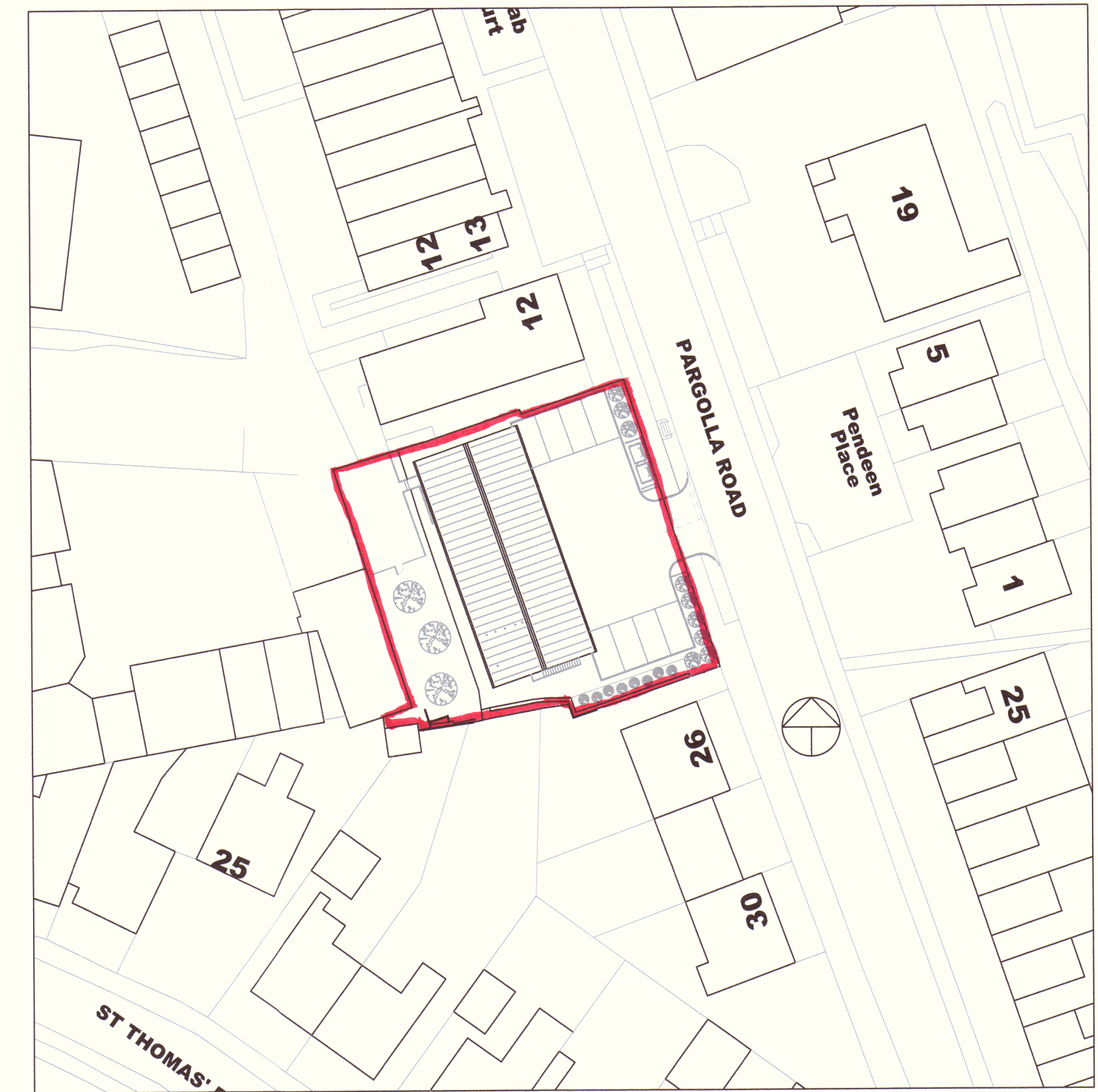
1:500 SITE PLAN
