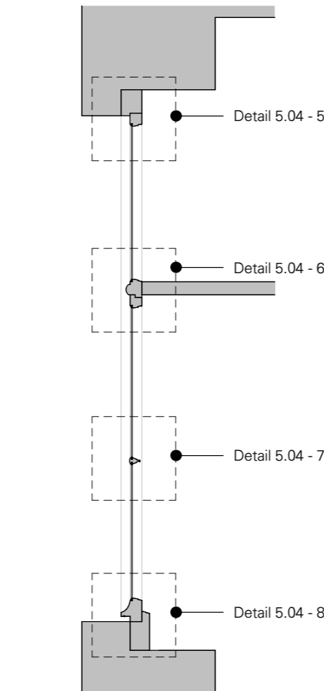
3 EXISTING SECTION 1 : 20
