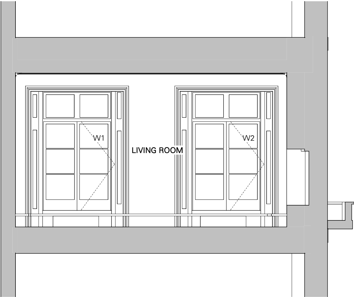
DD' EXISTING SECTION DD' 1 : 50
