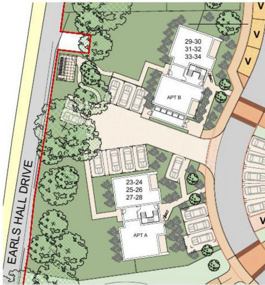
SITE PLAN 1:500
