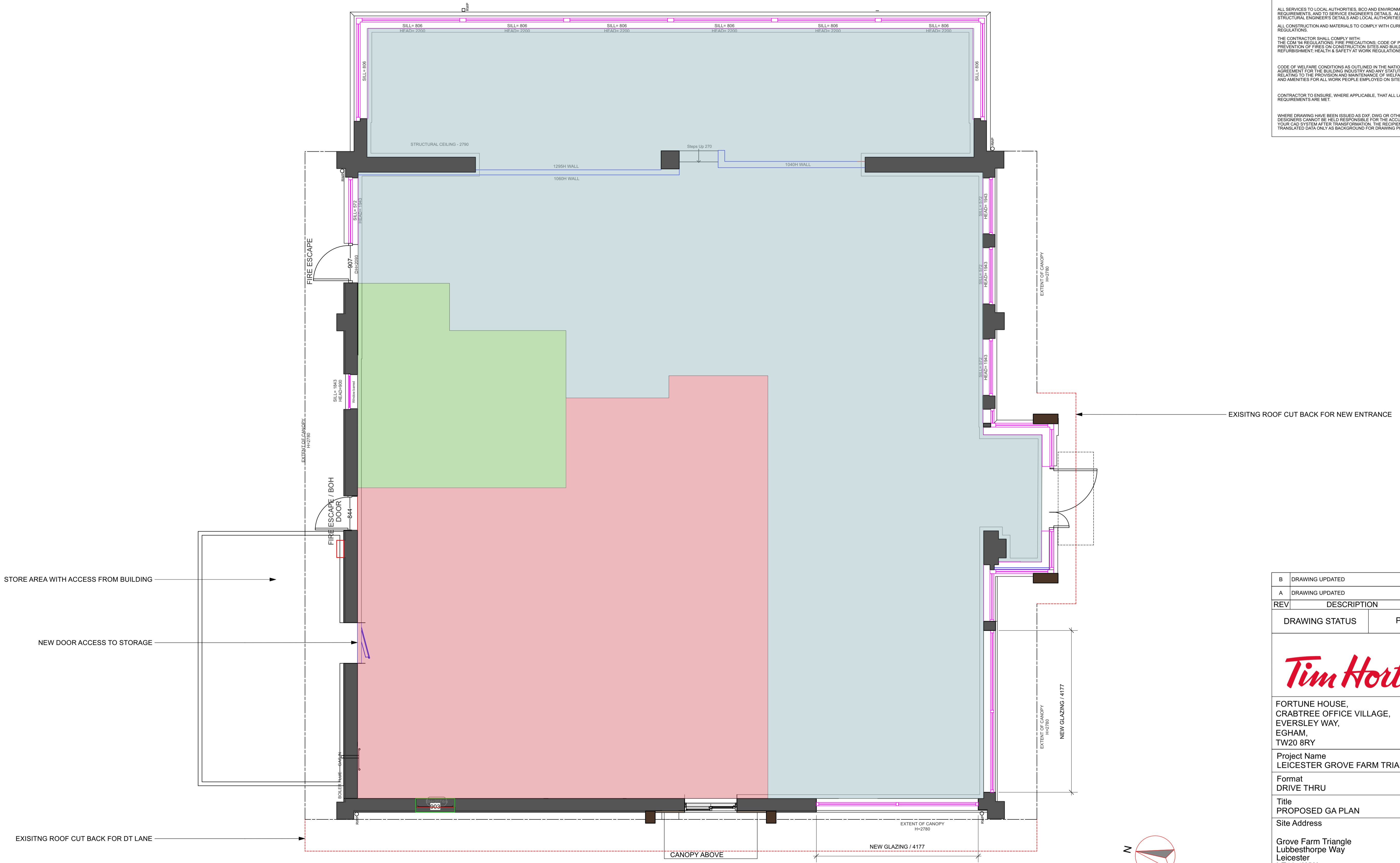
1 G FLR GA PLAN Scale: 1:50
