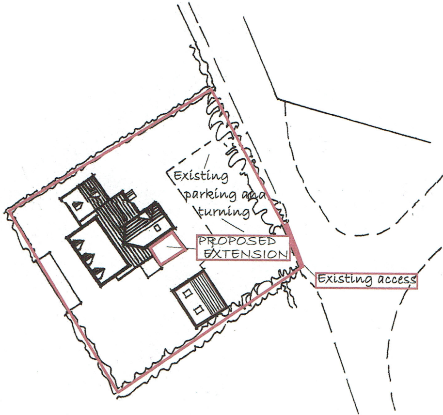
SITE PLAN 1:500
