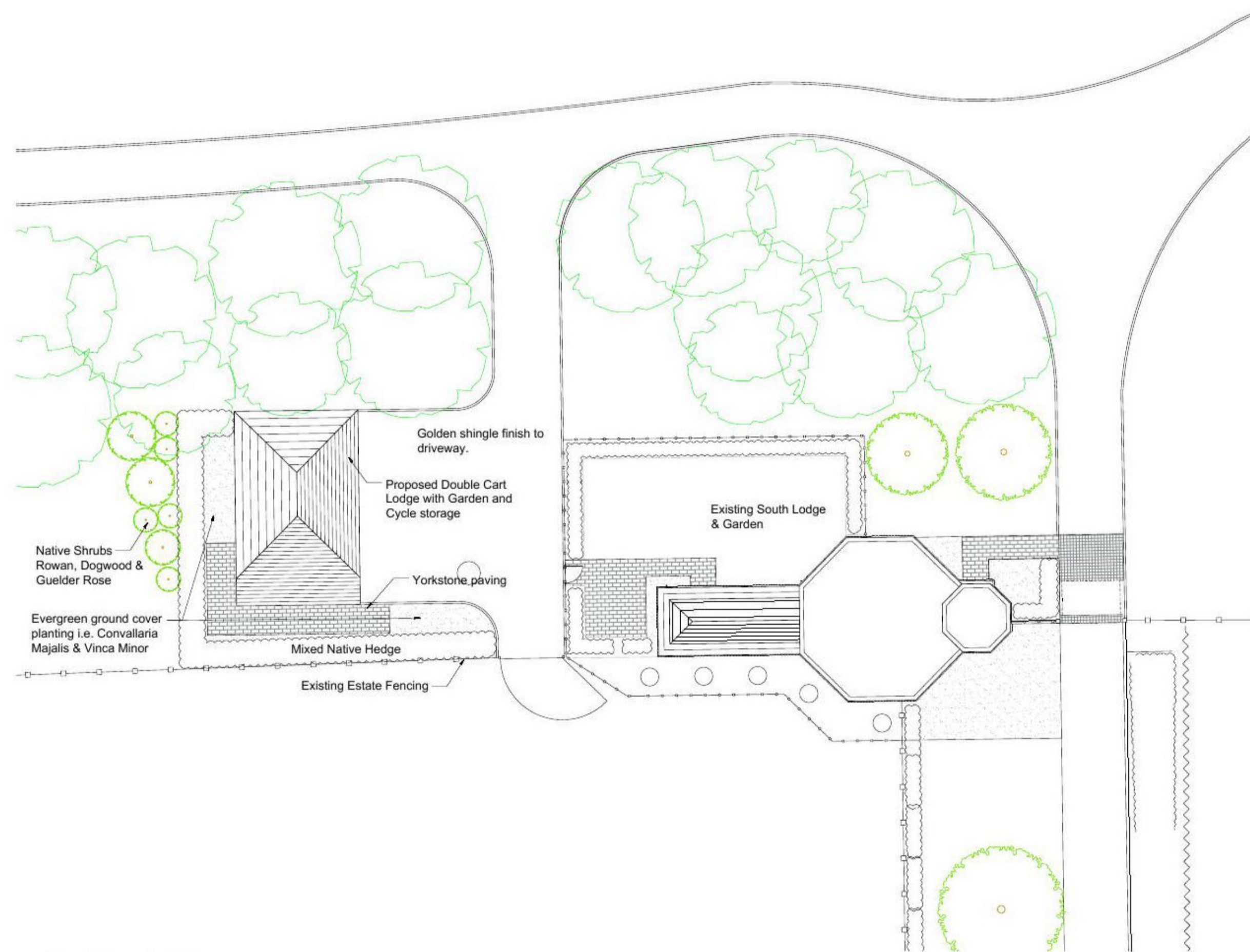
Site Plan 1:200
