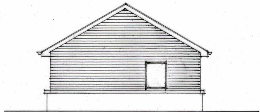
NE Elevation
