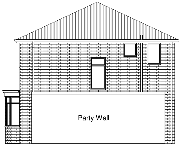
4 Side Elevation b-b 1 : 100
