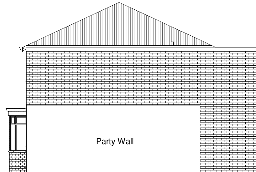
4 Side Elevation b-b 1 : 100
