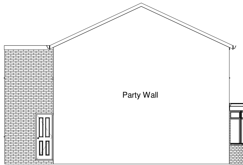
2 Side Elevation a-a 1 : 100
