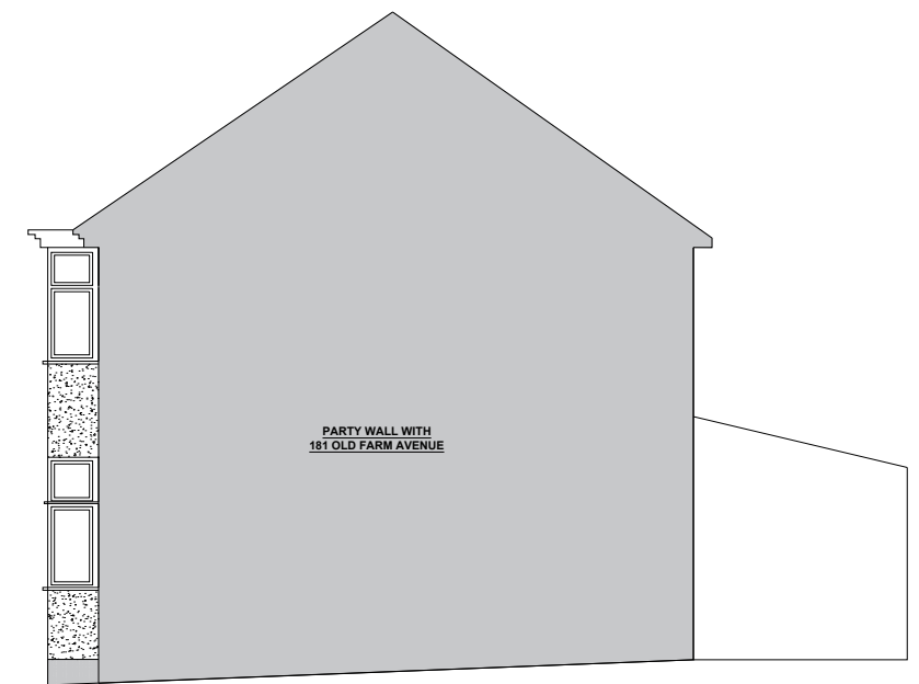
ELEVATION D-D
