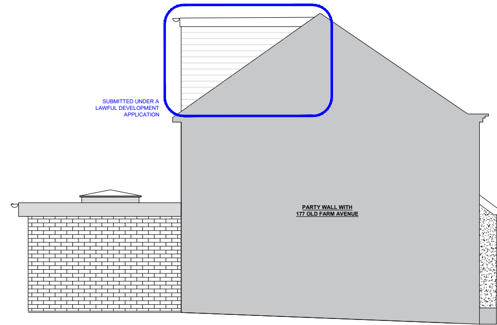
ELEVATION B-B
