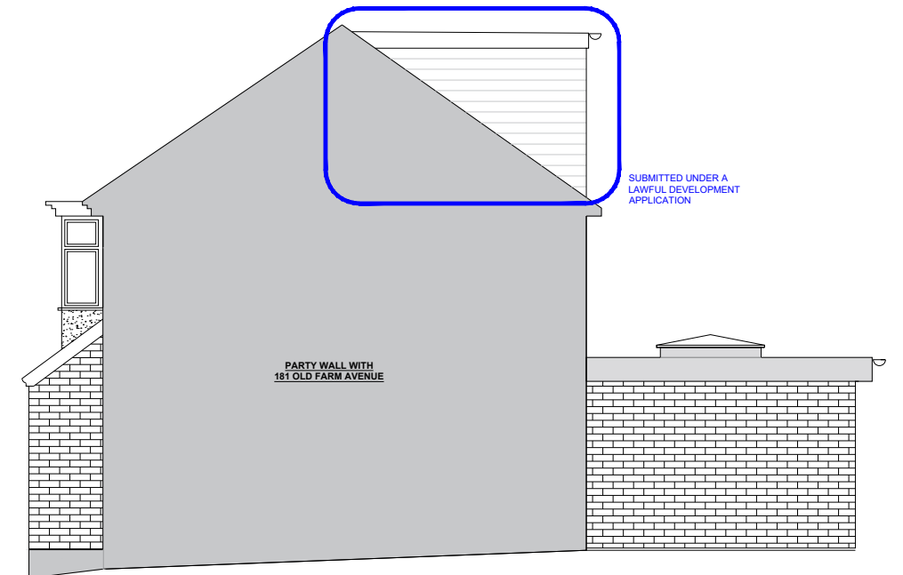
ELEVATION D-D
