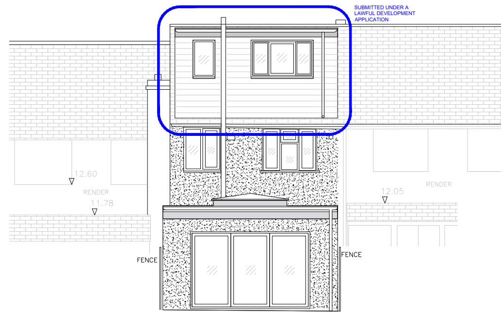
ELEVATION C-C
