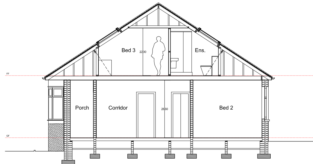
4 Section 1:100 @ A3
