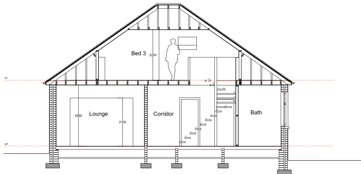
3 Section 1:100 @ A3
