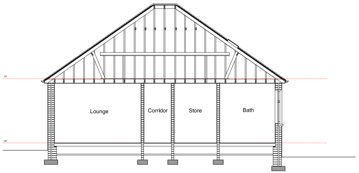
3 Section 1:100 @ A3
