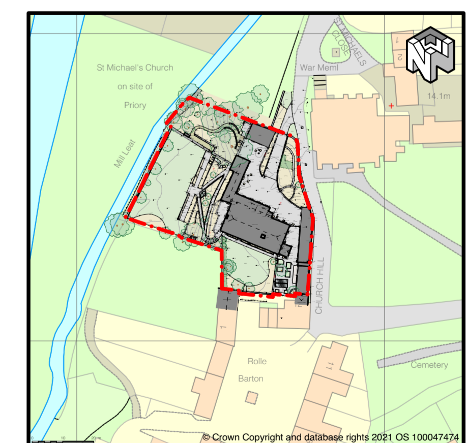
Site Plan 1:1250
