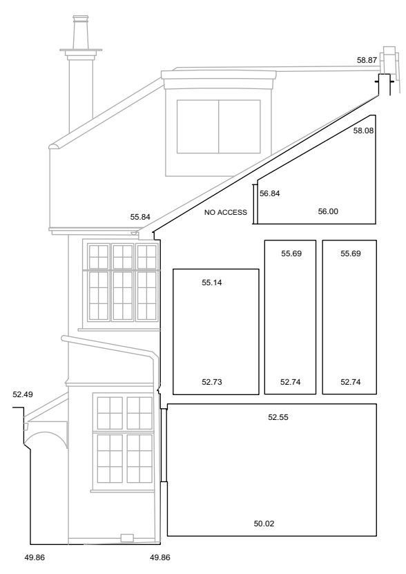
2 Existing Section DD Scale: 1:100
