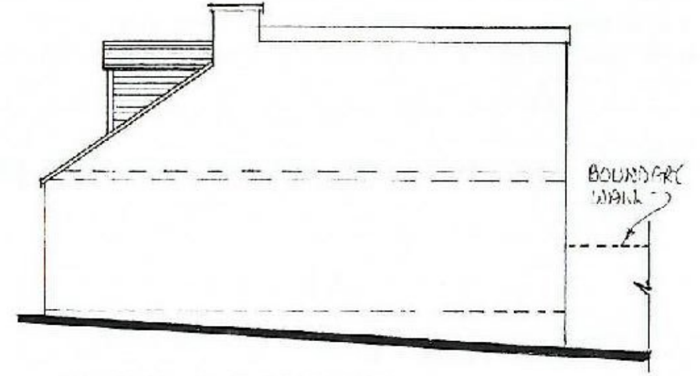
EXISTING N. E. ELEVATION.
