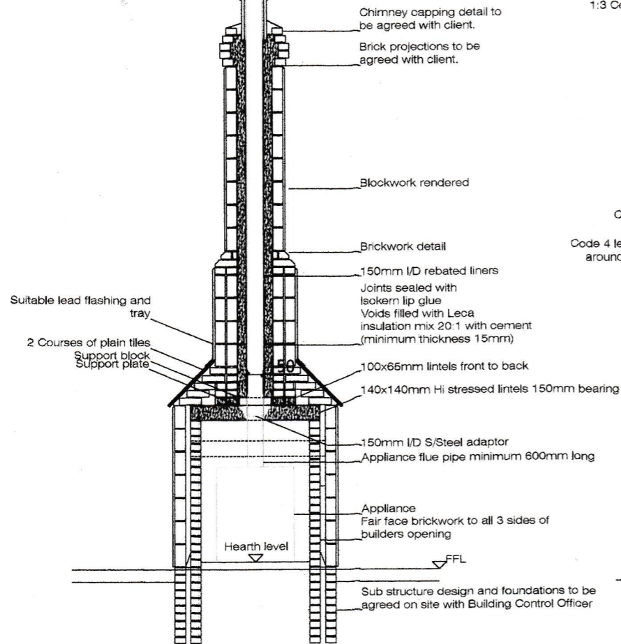
Section A-A
