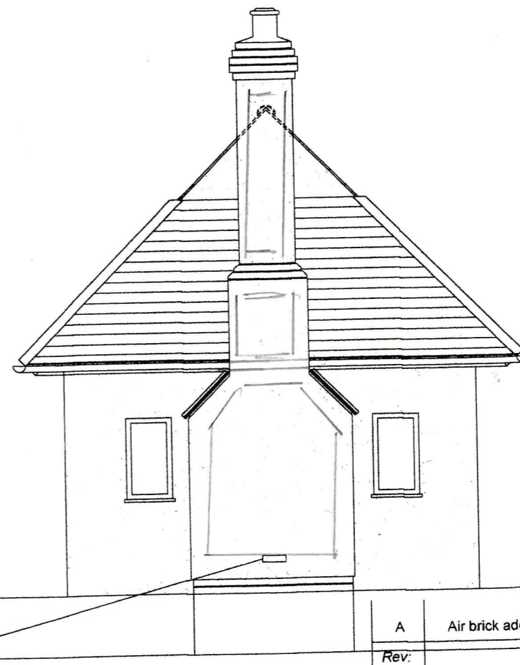
End elevation
