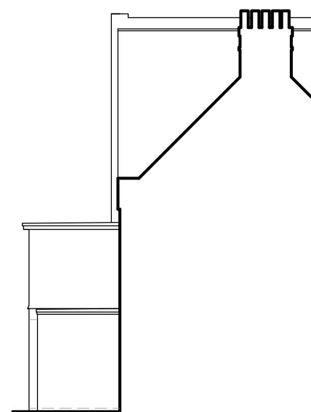
Flank elevation 1:100
