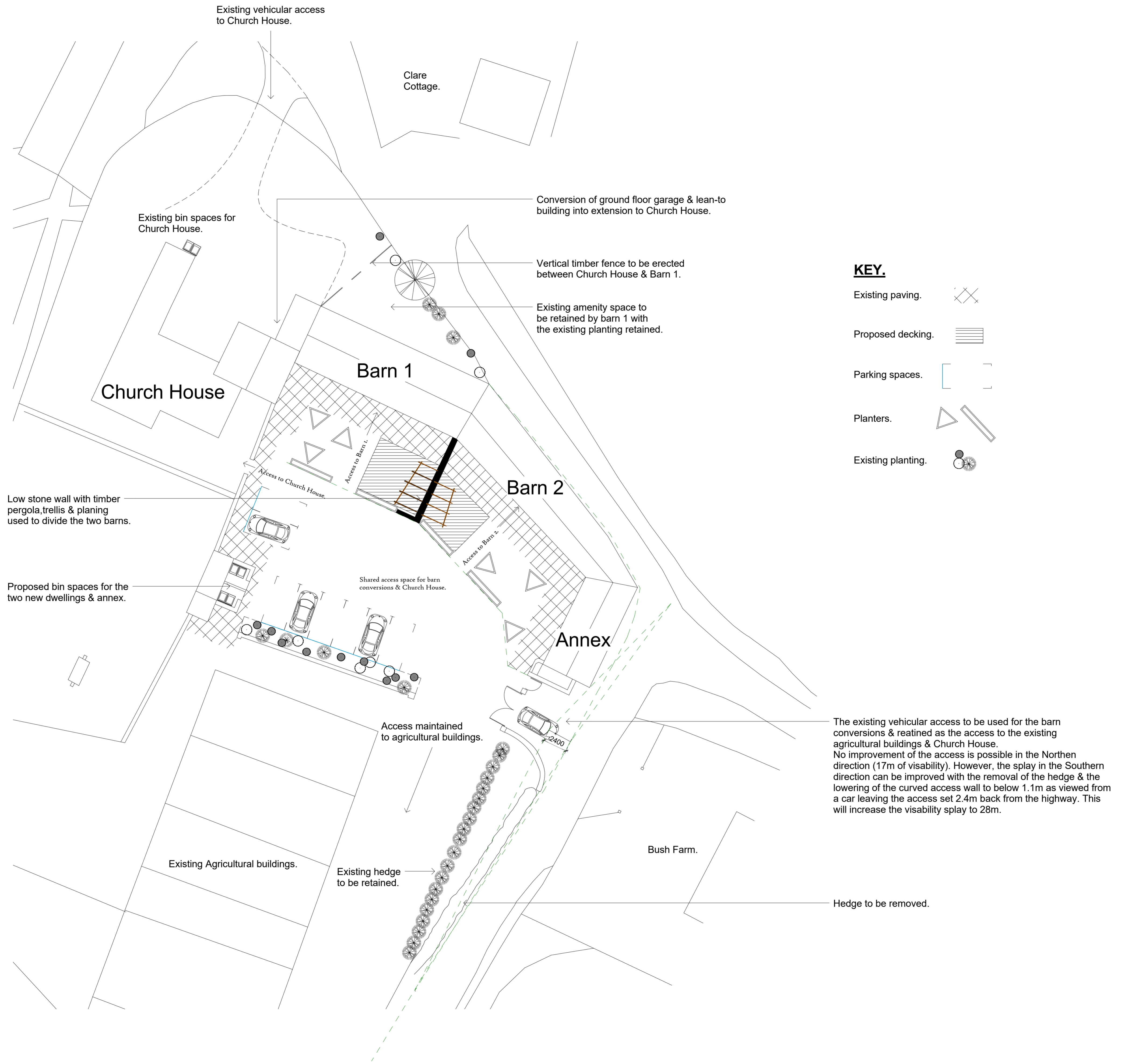
Block Plan 1 : 200
