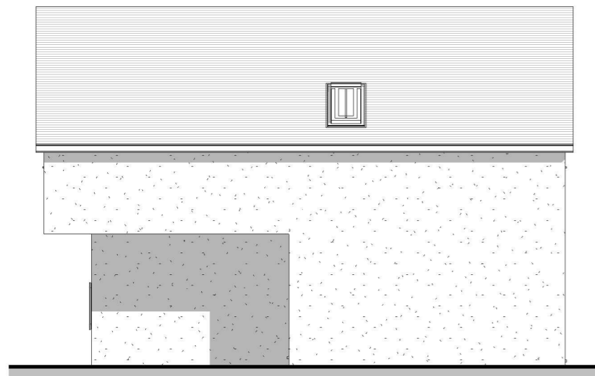
Side 1 1 : 100
