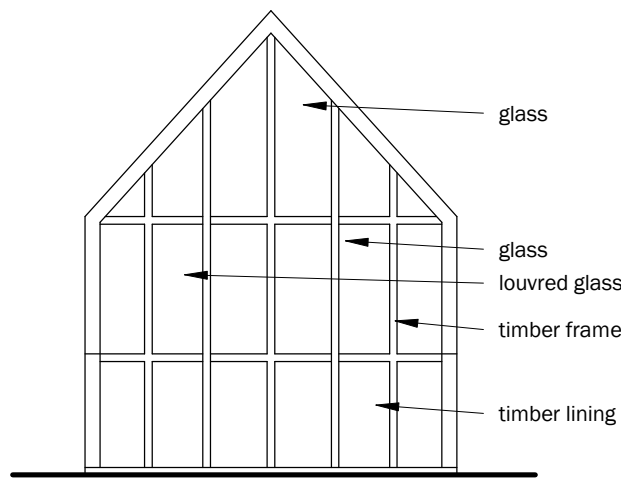
NE ELEVATION
