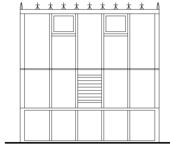
SE ELEVATION
