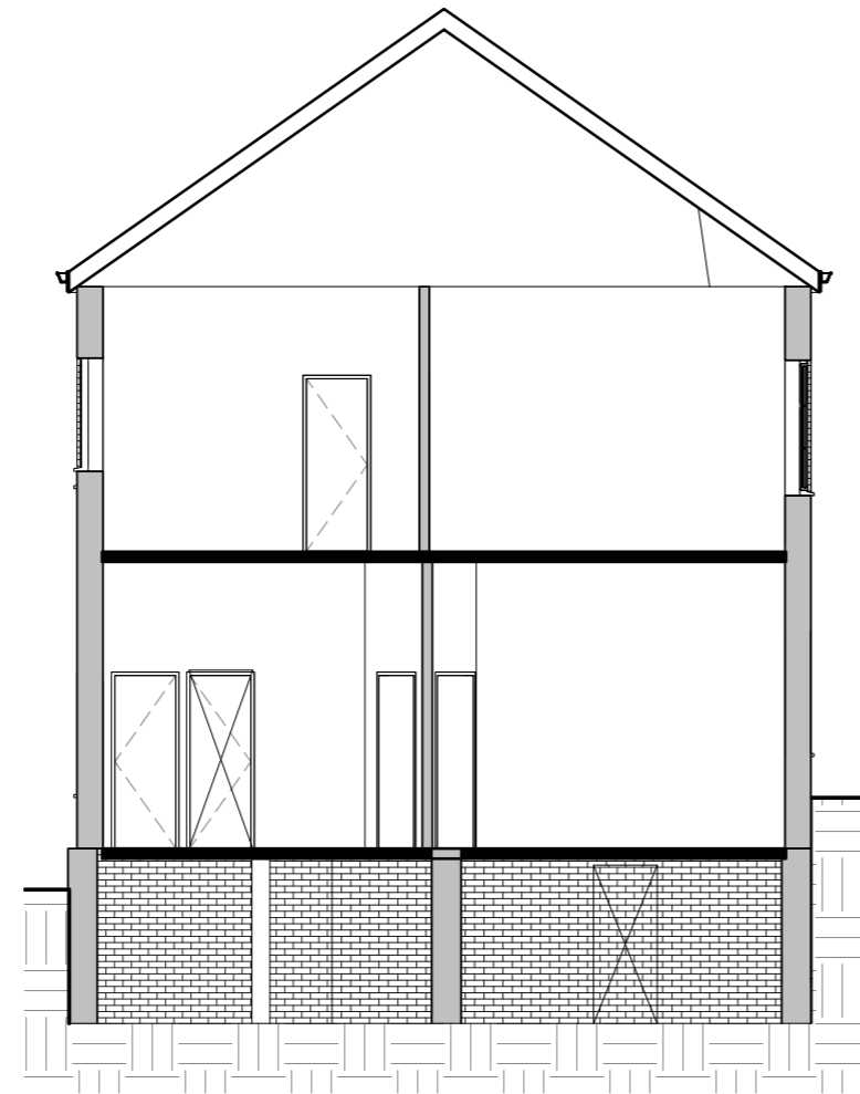
1 Section Existing 1 : 100
