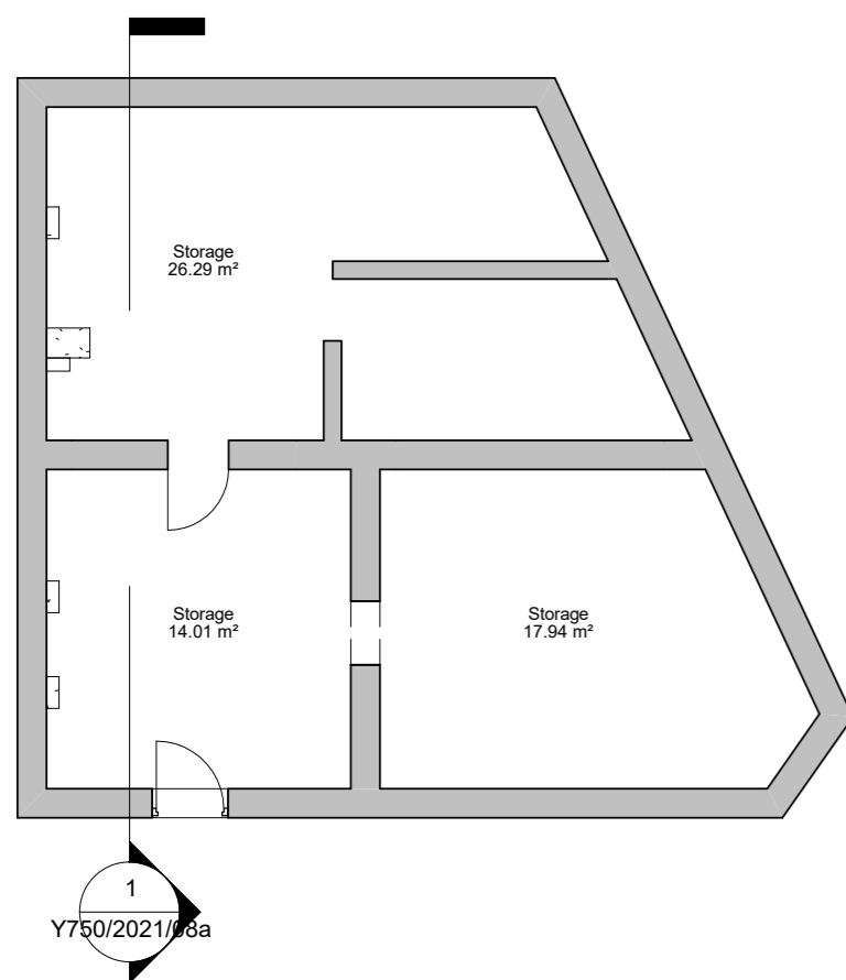
1 00. Basement Existing 1 : 100
