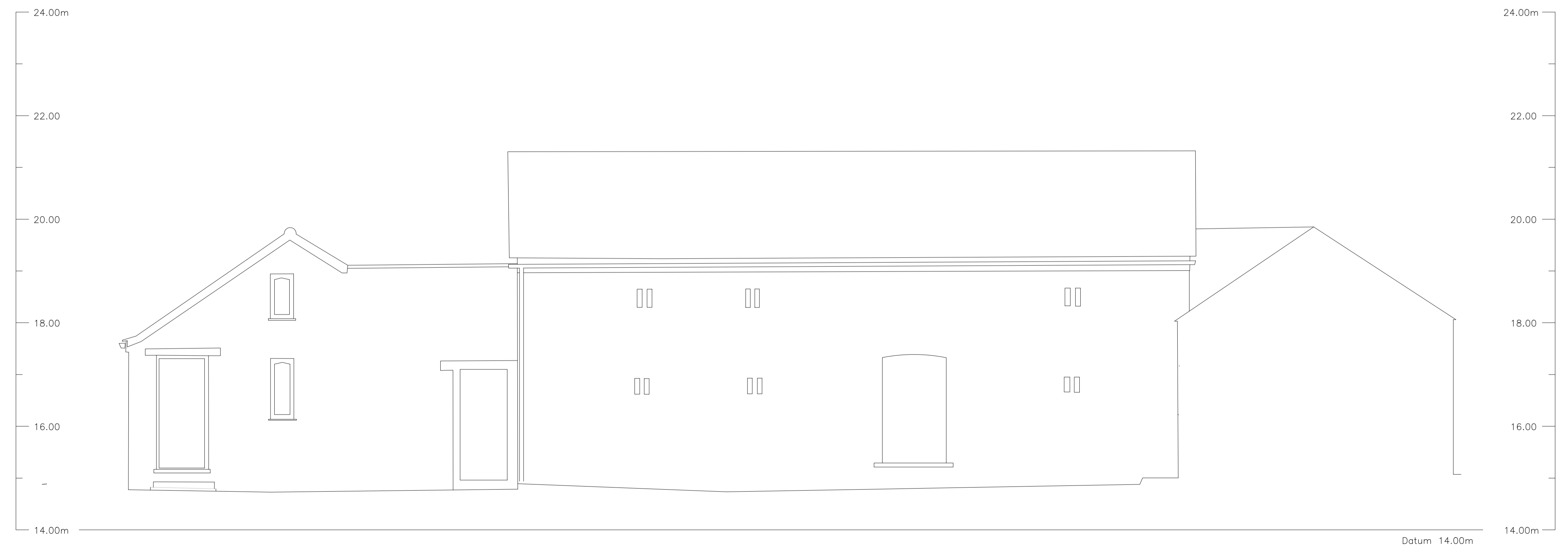
EXISTING ELEVATION 02
