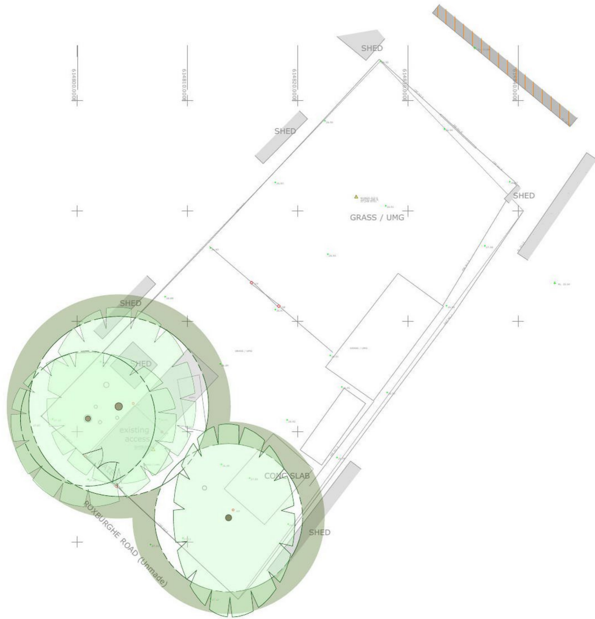
SITE PLAN 1:200
