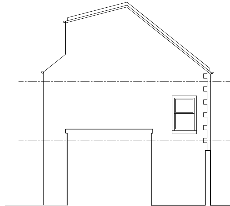
SIDE ELEVATION (S.W.)
