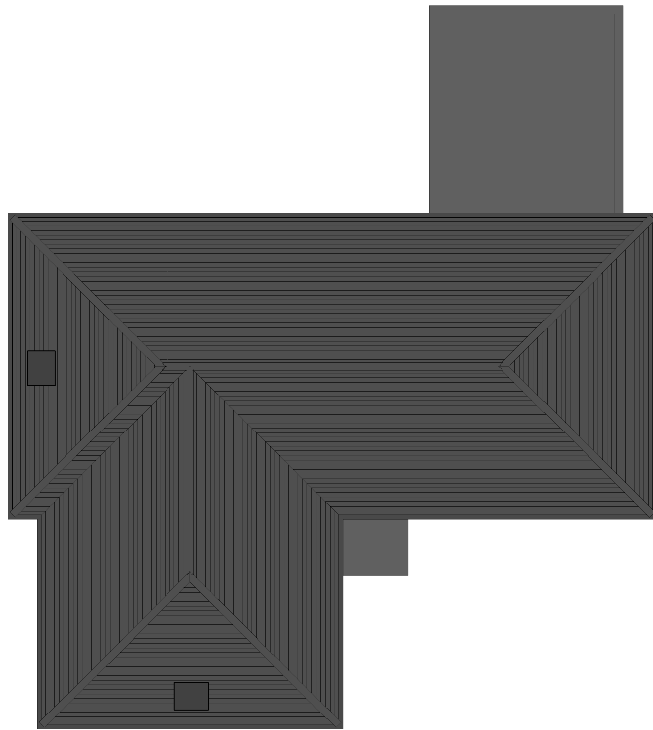
1 Roof Plan 1 : 100
