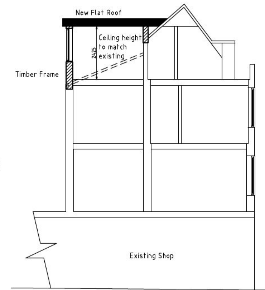
Section A-A 1:100
