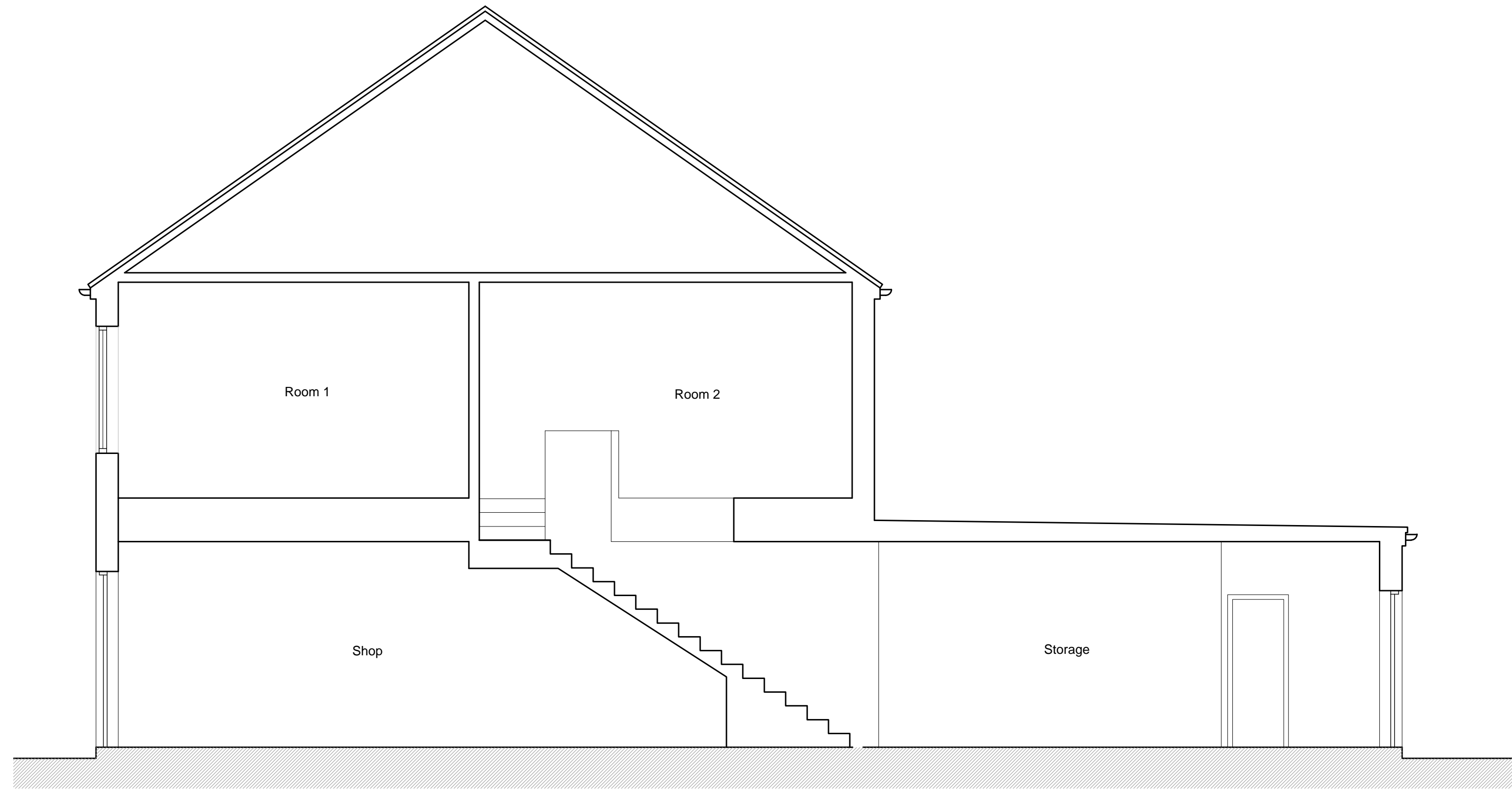
Section A-A
