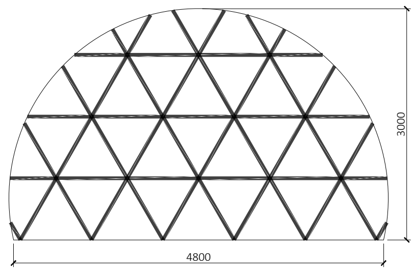
ELEVATION
